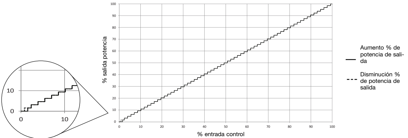
Modo 2: Conmutación de 1 ciclo completo
